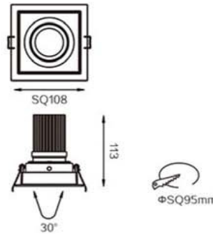
FS5047A-13 Max. 13W
