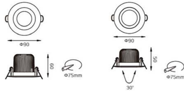
FS1008-09 / FS1007-09 Max.9W
